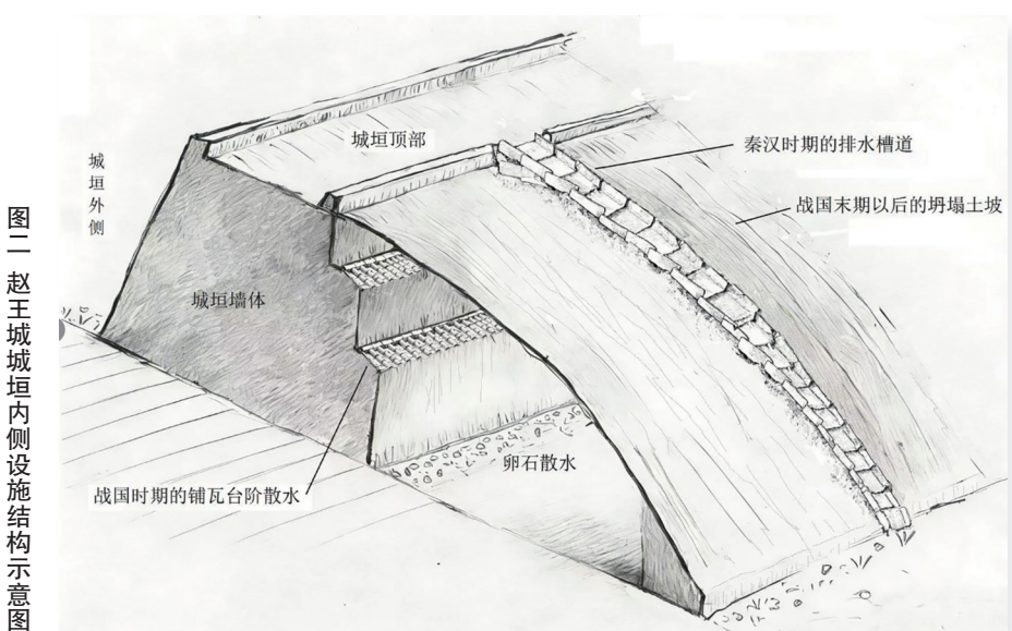
图二 赵王城城垣内侧排水设施结构示意图
