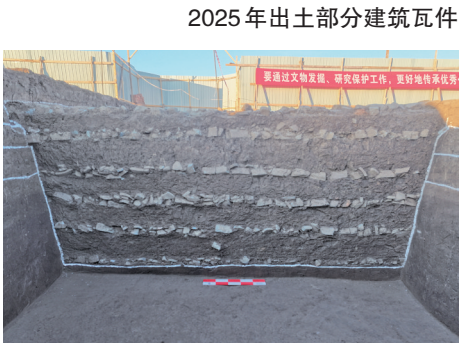
F1 西墙基剖面照
